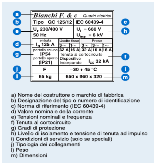
Figura 13.2 – Esempio di targa dei quadri ASC
