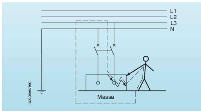
Figura 6.2 – Contatto indiretto
